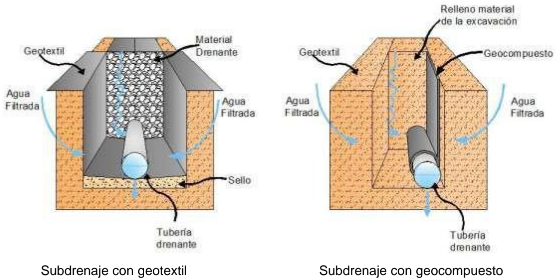
Figura 605-01 Sistemas de Subdrenajes
